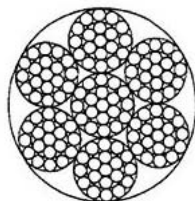
6x19+IWS
