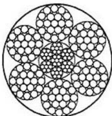
6x19+IWR
