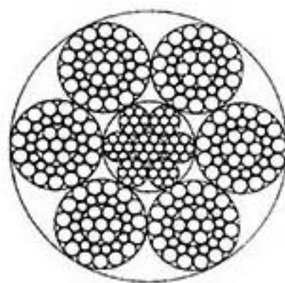
6x37S+IWR
