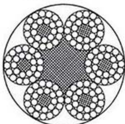
6x24+7FC
