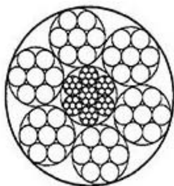
6x7+IWR
