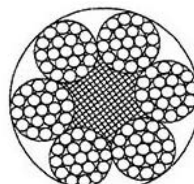
6x19+FC
