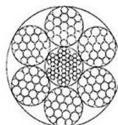
6x19W+IWR
