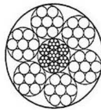
6x7+FC
