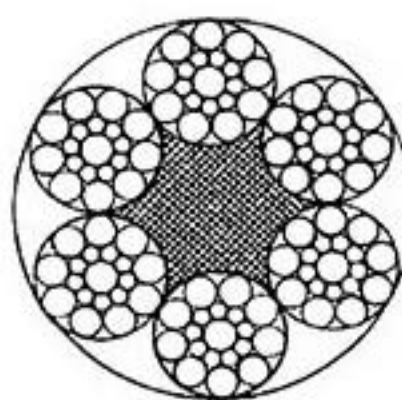
6x19S+FC
