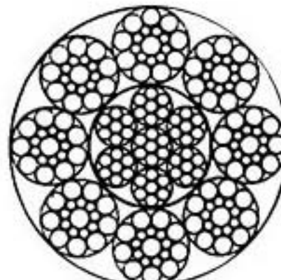
8x19S+IWR
