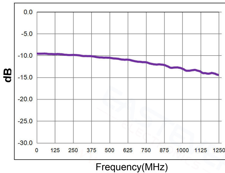
Port 1 Return Loss(pin2)
