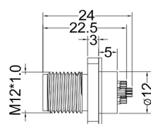
12pin
