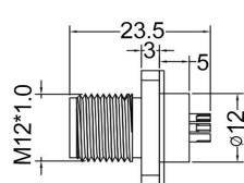
5pin
